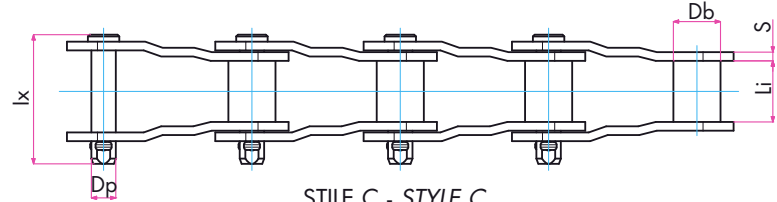
STILE C - STYLE C
