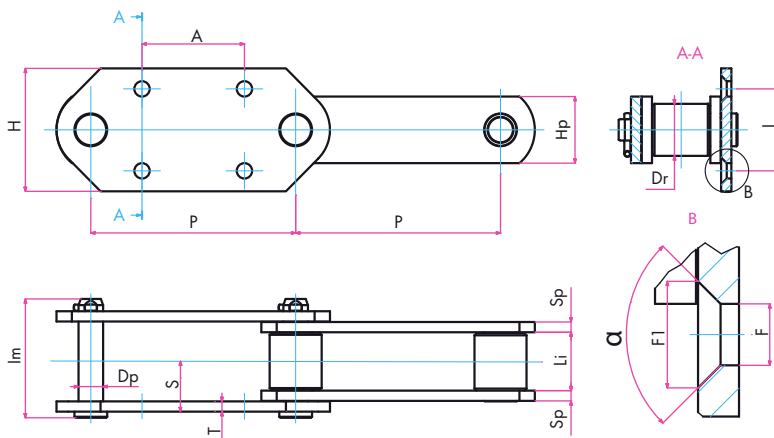
STILE G4-1 / STYLE G4-1
