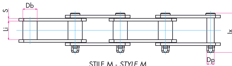
STILE M - STYLE M
