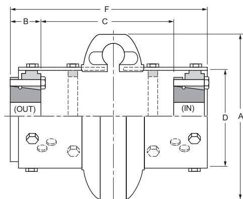
QD
