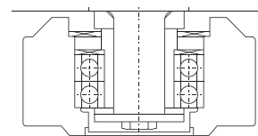
Пример конструкции уплотнения внешнего ролика (проверенная надежность более 15 000 часов)
