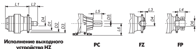
Конструкция А 300 - 307
