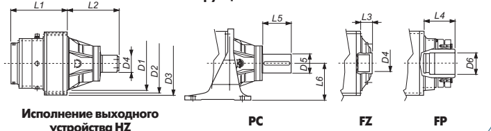
Конструкция В 309 - 321
