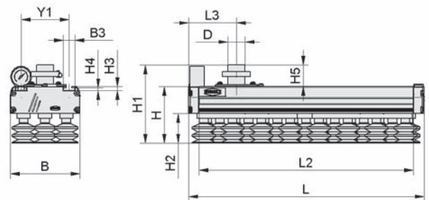
FMP SPB2
