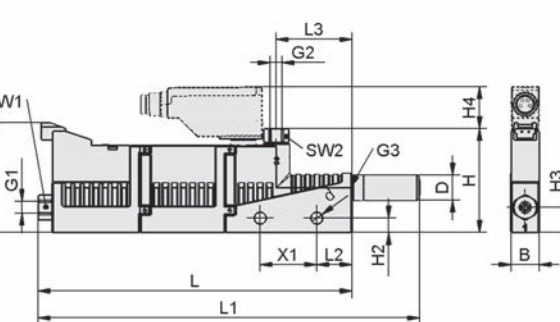
SBP-C 05/07 G01 NC AI (VS-T)
