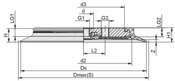
SPU 125 - 210 AE
