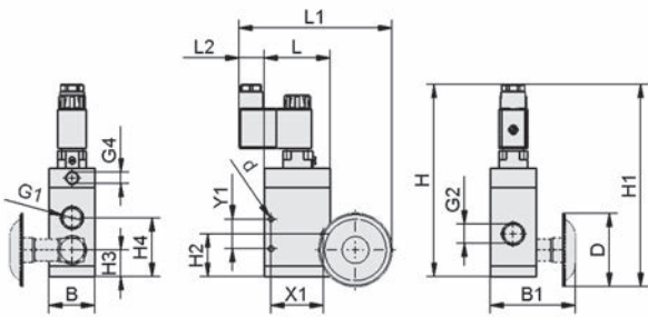
EMVP 10
