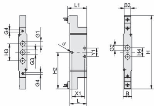
EMVP 5 - 8 IMP
